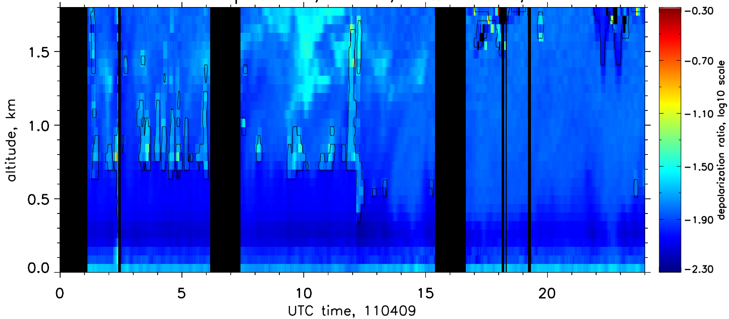
Volume linear depol. ratio, 532nm, res.: 10 min., 60–60 m
