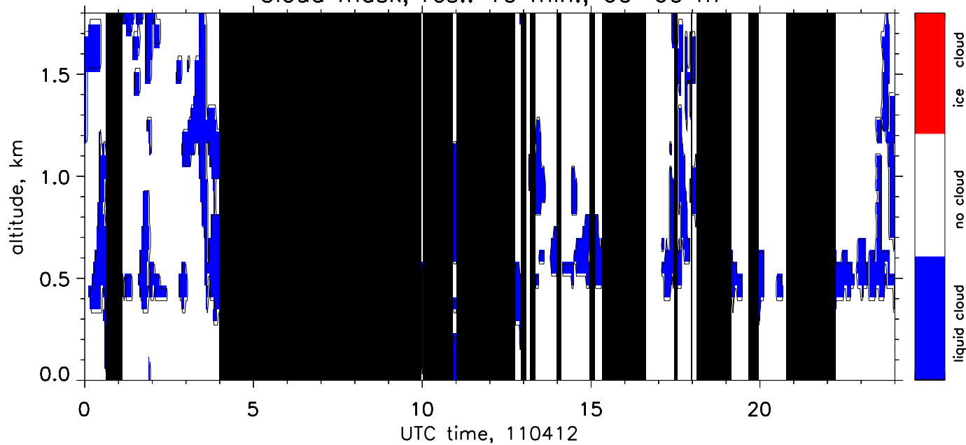
Cloud mask, res.: 10 min., 60–60 m
