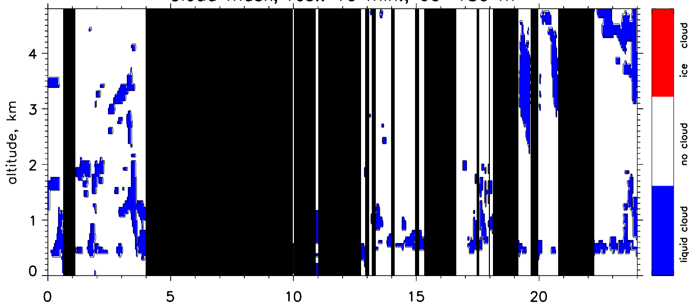
Cloud mask, res.: 10 min., 60–180 m
