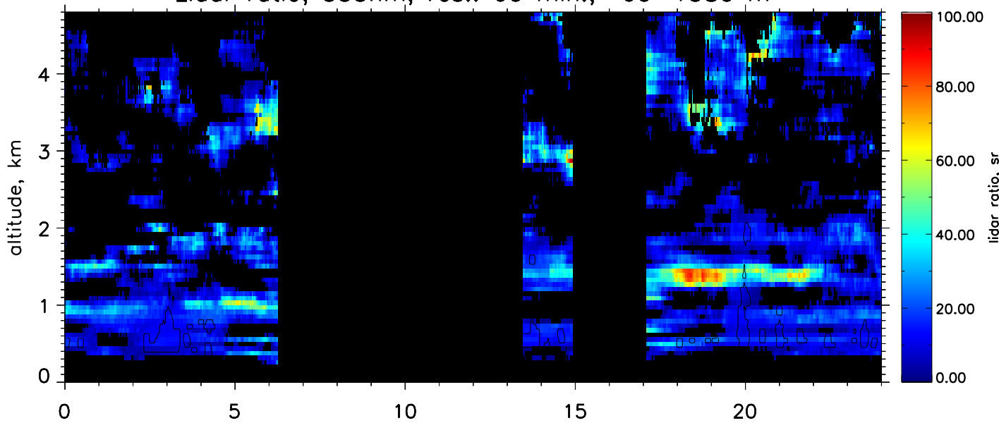
Lidar ratio, 355nm, res.: 60 min., 60–1380 m
