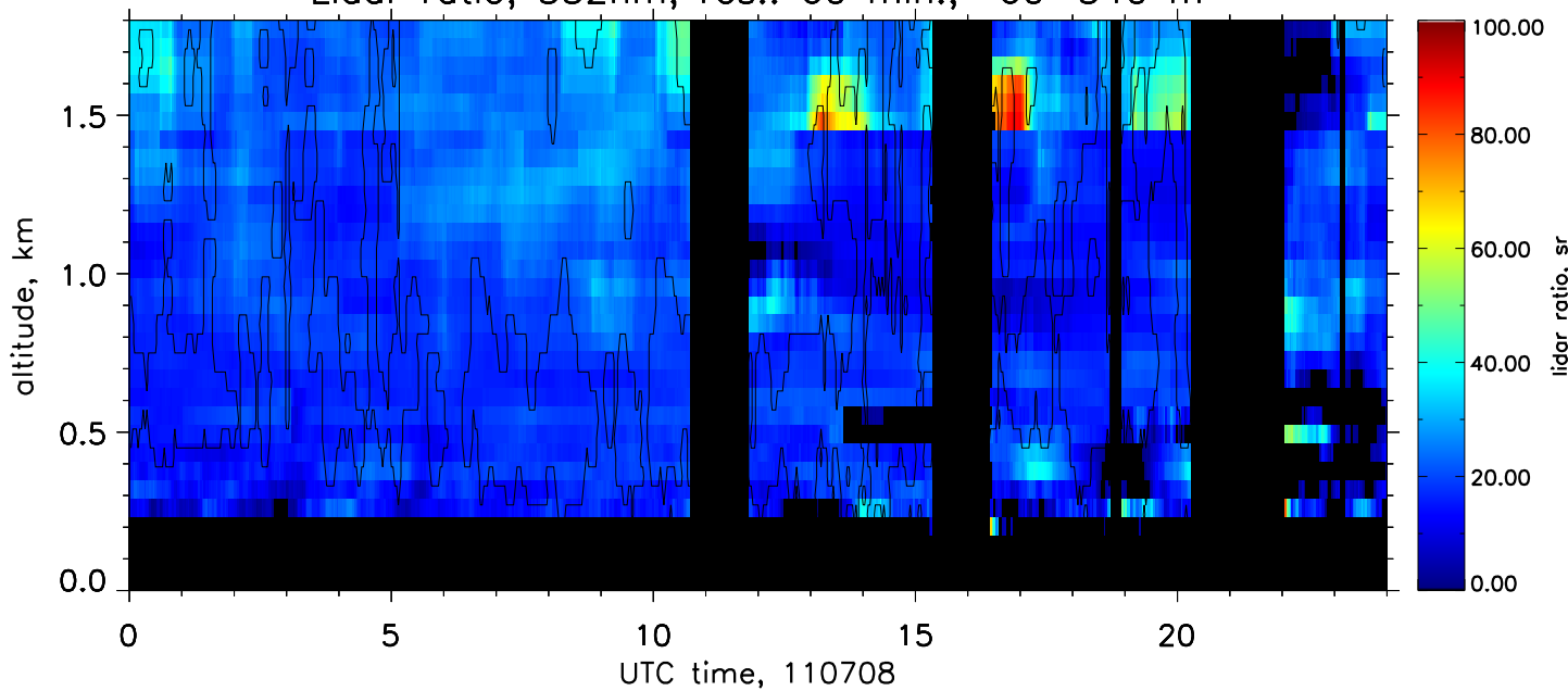
Lidar ratio, 532nm, res.: 60 min., 60–540 m
