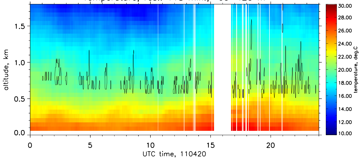
Temperature, res.: 118 min., 60–420 m
