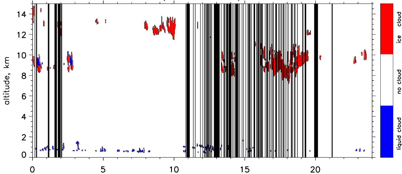
Cloud mask, res.: 2 min., 60–660 m
